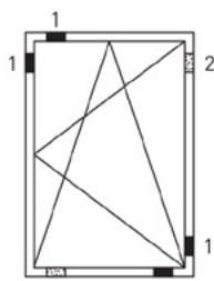
Поворотно-откидная створка
